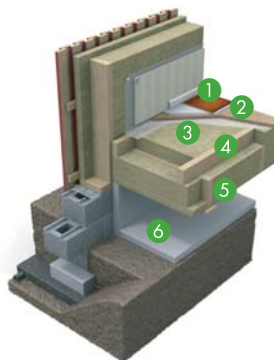
Конструкция нижнего каркасного перекрытия
