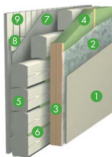
Конструкция с внутренним каркасным утеплением
