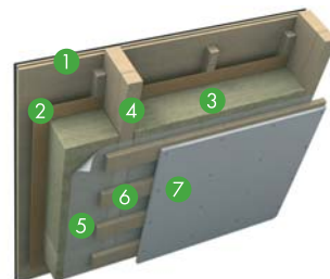
Конструкция кровельного каркасного перекрытия
