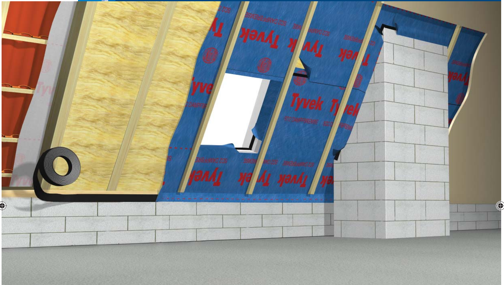
Рис. 10 Монтаж пароизоляции
