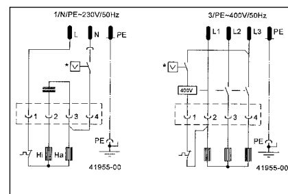
Δ-соединение для, низкое напряжение
