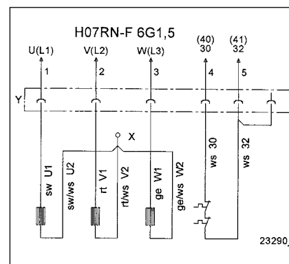
Y-koppling för hög spänning
