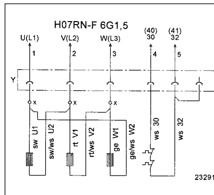
Δ-koppling för låg spänning
