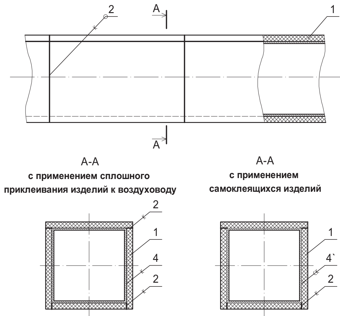
Рис. 15. Тепловая изоляция воздуховодов систем вентиляции и кондиционирования с помощью изоляционных листов марок Armaflex ACE и Armaflex XG в различных вариантах в обычном и в самоклеящемся исполнении, с покрытием и без покрытия), при расположении внутри помещения. Без применения самоклеящейся ленты.
