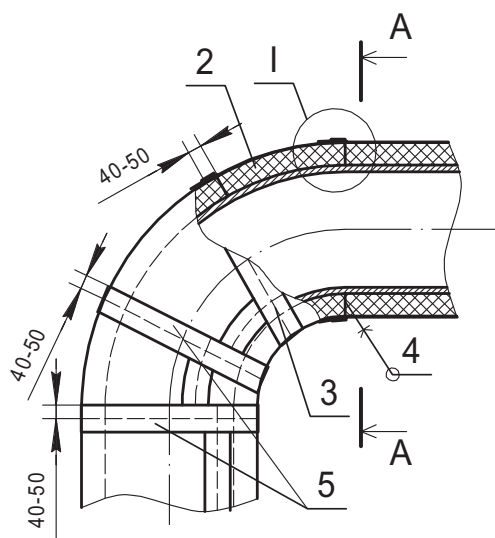
Рис. 22. Тепловая изоляция отвода трубопровода с помощью изделия, раскроенного и склеенного из листов (рулонов) "ARMAFLEX" для труб 89 \text{ мм} \leq D_n \leq 500 \text{ мм} , с отдельно установленным покрытием марки Arma-Chek D или Arma-Chek Silver при расположении в помещении (с применением самоклеящихся лент для покрытия).
