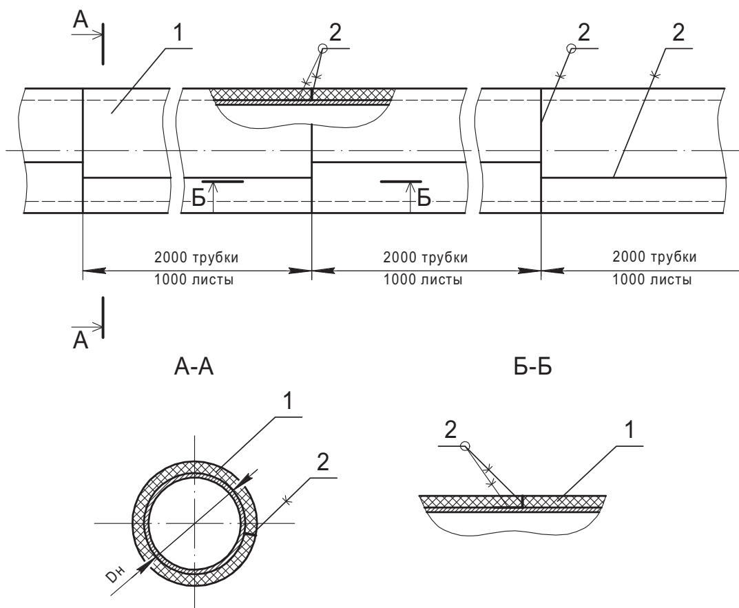
Рис. 1. Тепловая изоляция трубопровода с помощью изоляционных изделий "ARMAFLEX" (без применения самоклеящейся ленты), для труб с Дн менее 600 мм
