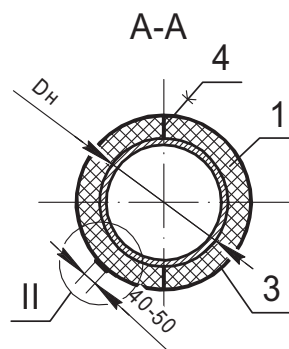
Рис. 22. Тепловая изоляция отвода трубопровода с помощью изделия, раскроенного и склеенного из листов (рулонов) "ARMAFLEX" для труб 89 \text{ мм} \leq D_n \leq 500 \text{ мм} , с отдельно установленным покрытием марки Arma-Chek D или Arma-Chek Silver при расположении в помещении (с применением самоклеящихся лент для покрытия).
